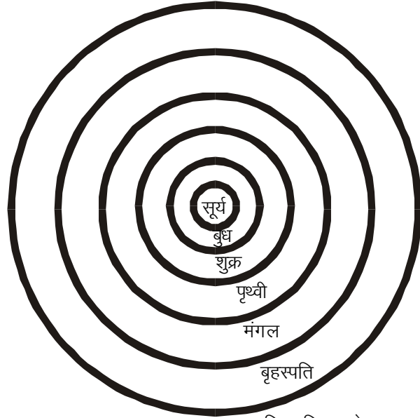
चित्र 7 शनि, यूरिनस, नेप्चून, प्लूटो
